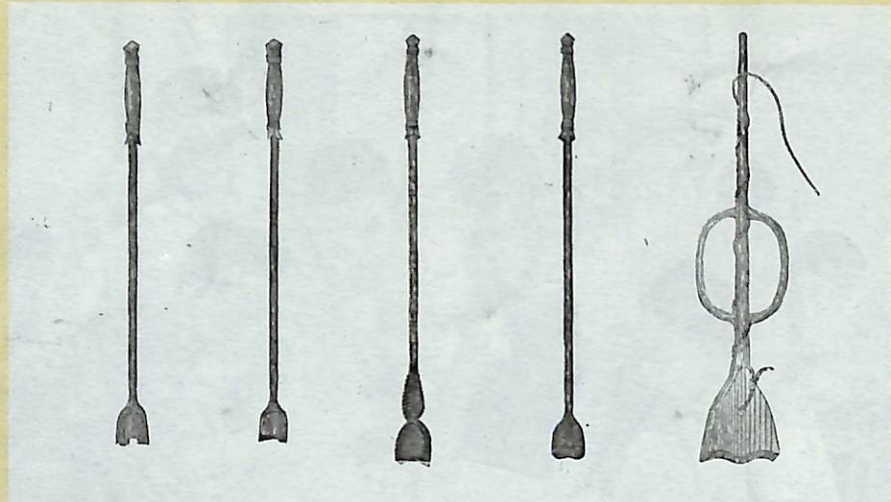
清代（公元一六四四——一九一一年）凿井用的各种钻头。（原载清代《四川盐法志》）
